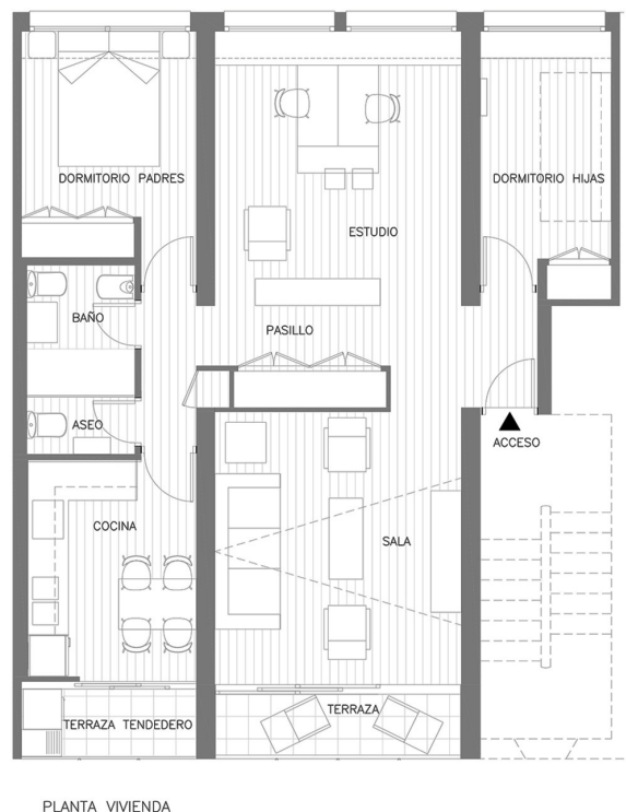
PLANTA VIVIENDA
